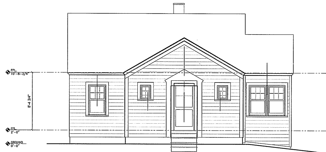
4 WEST ELEVATION SCALE: 1/8" = 1'-0"
