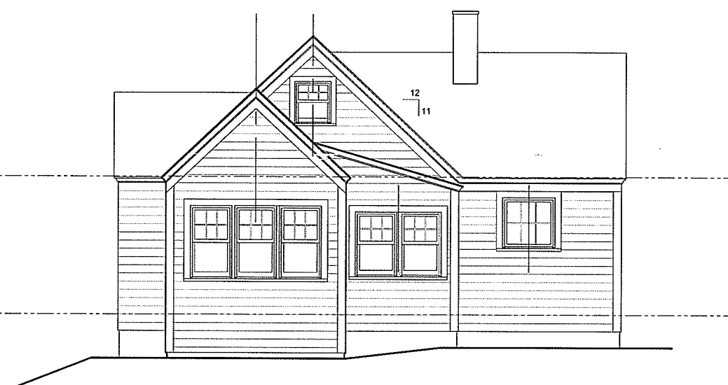
3 SOUTH ELEVATION SCALE: 1/8" = 1'-0"
